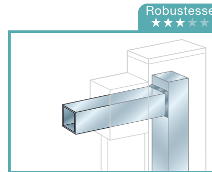
Inox soudé intégré invisible Cadre 30 x 30 mm ou 50 x 30 mm suivant dimension
