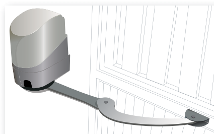
▲ Bloc moteur avec armoire de gestion intégrée
