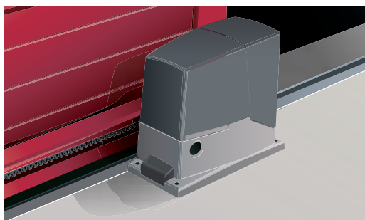
Bloc moteur avec armoire de gestion
